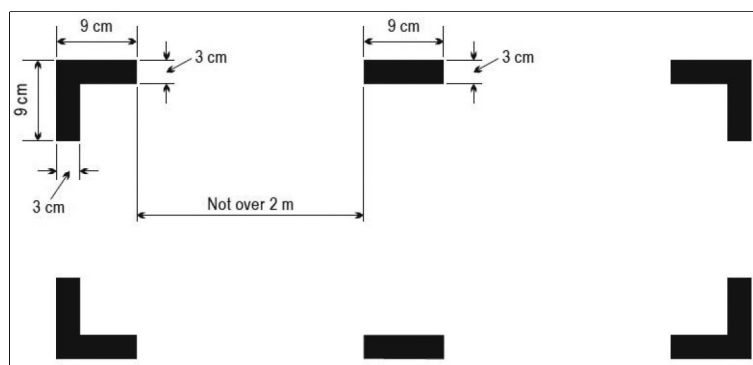
Figura 1. Vijëzimi i pikave të hyrjes me thyerje nga jashtë (në rast emergjence)
