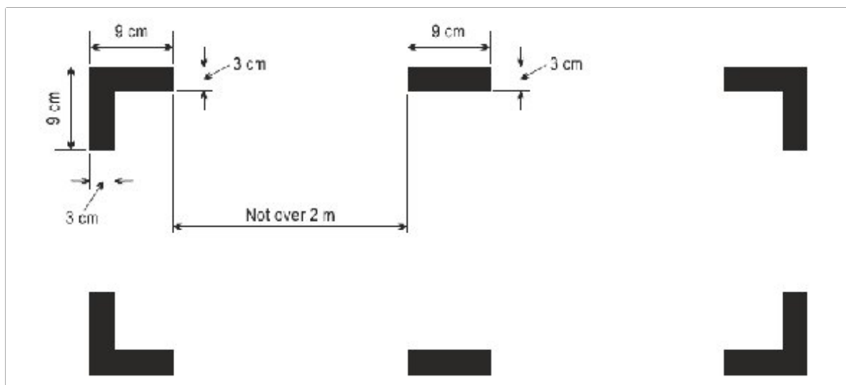
Figura 1. Vijëzimi i pikave të hyrjes emergjente me thyerje
