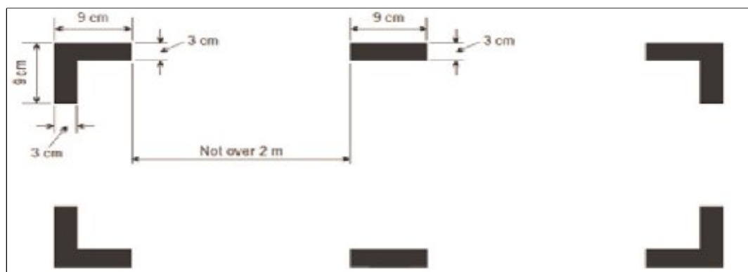
Figura 1. Skema e pikave të hyrjes me thyerje
