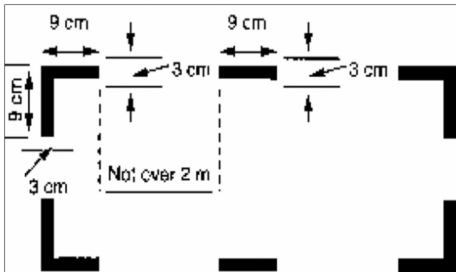
Figura 1. Shënjimi i pikave të hyrjes
