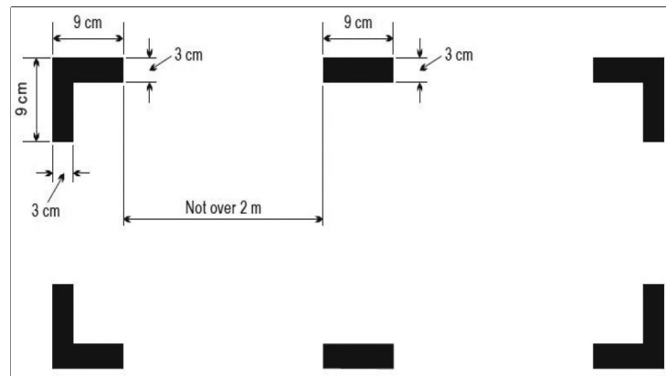
Figura 1. Shënimi i pikave të hyrjes me thyerje
